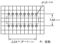
印刷基板加工尺寸 (TOP VIEW)
